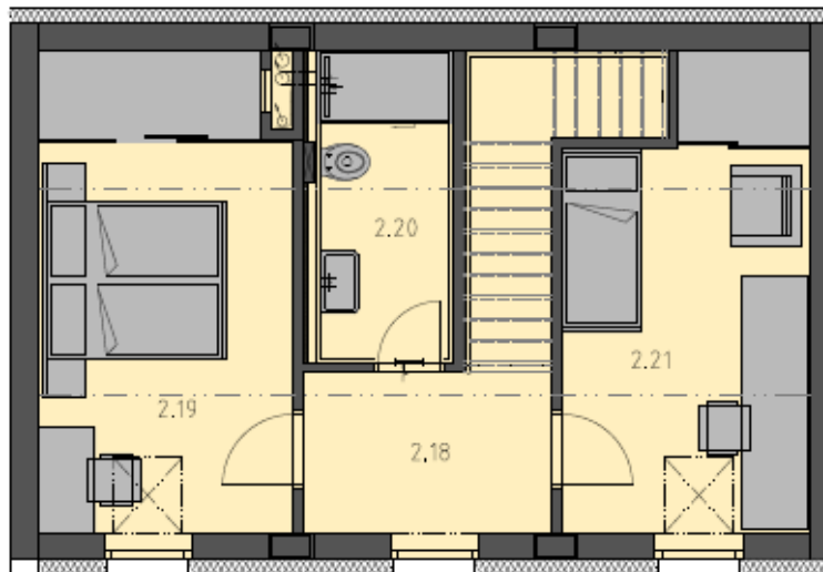
PŮDORYS 2.NP:
